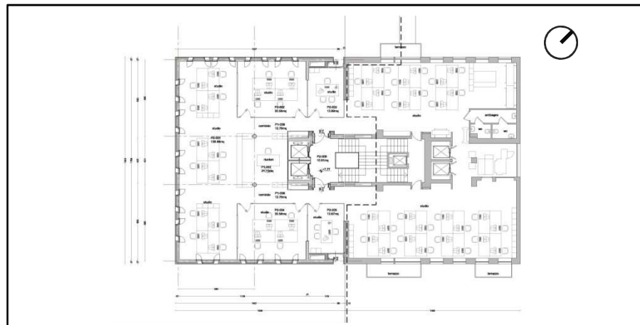
Pianta piano tipo
