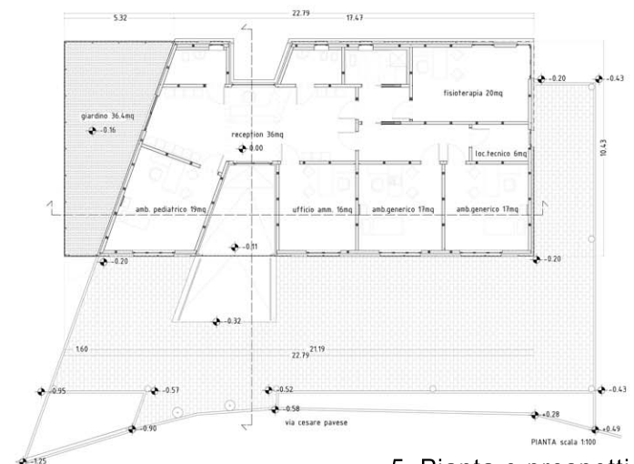
5_Pianta e prospetti
